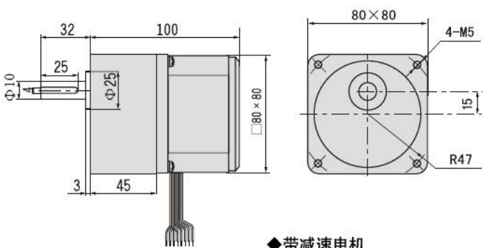
带减速电机
