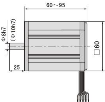
电机
