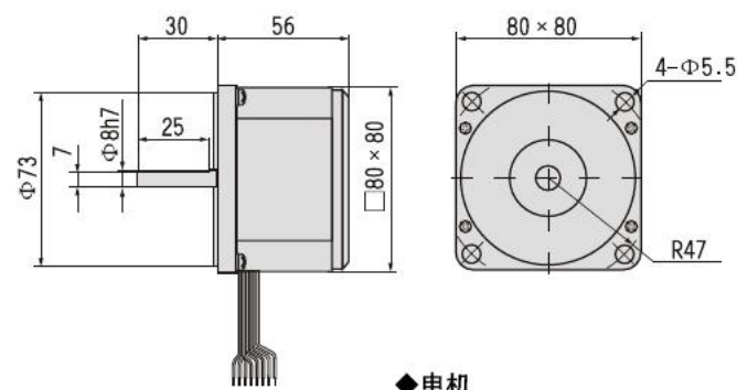
电机
