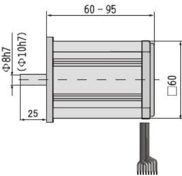
电机
