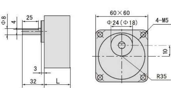
减速箱
