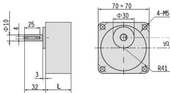
减速箱
