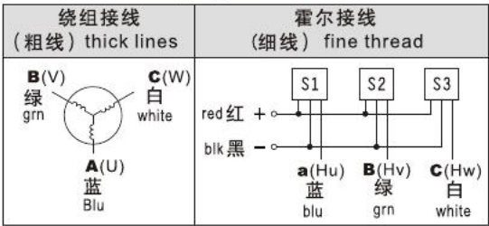
◆接线方式: Wiring diagram
